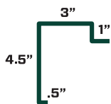
SLIDING DOOR TRIM A
