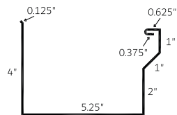
Eavestrough 6" (ET 6)
