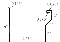
Eavestrough 5" (ET 5)
