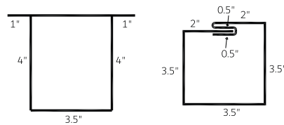
Eavestrough Outlet 5" and 6" (ETO)
