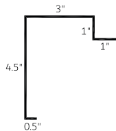
Sliding Door Trim 'A' 3/4" (SDA 0.75)
