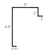
Sliding Door Trim 'A' 3/4" (SDA 0.75)
