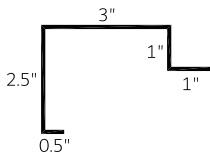
Sliding Door Trim 'B' 3/4" (SDB 0.75)
