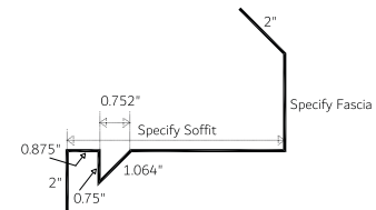
Eavestrough 6" (ET 6)
