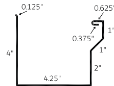
Eavestrough 5" (ET 5)
