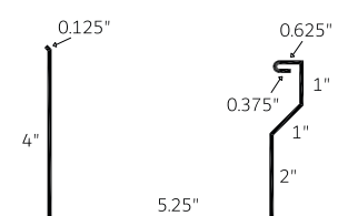
Eavestrough 6" (ET 6)
