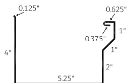
Eavestrough 6" (ET 6)
