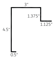
Sliding Door Trim 'A' 1-1/4" (SDA 1.25)
