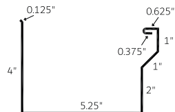
Eavestrough 6" (ET 6)
