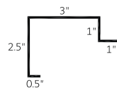
Sliding Door Trim 'B' 3/4" (SDB 0.75)
