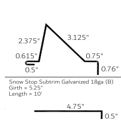
Legacy Snow Stop (LSNO)
