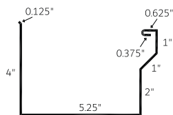
Eavestrough 6" (ET 6)
