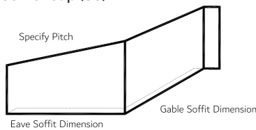
Corner Cap (CC)
