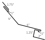
Legacy Under/Over 1" (LUOF 1)
