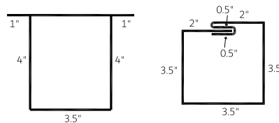
Eavestrough Outlet 5" and 6" (ETO)
