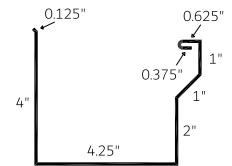
Eavestrough 5" (ET 5)
