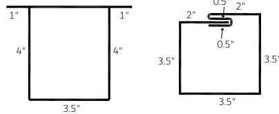
Eavestrough Outlet 5" and 6" (ETO)
