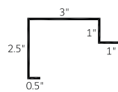
Sliding Door Trim 'B' 3/4" (SDB 0.75)
